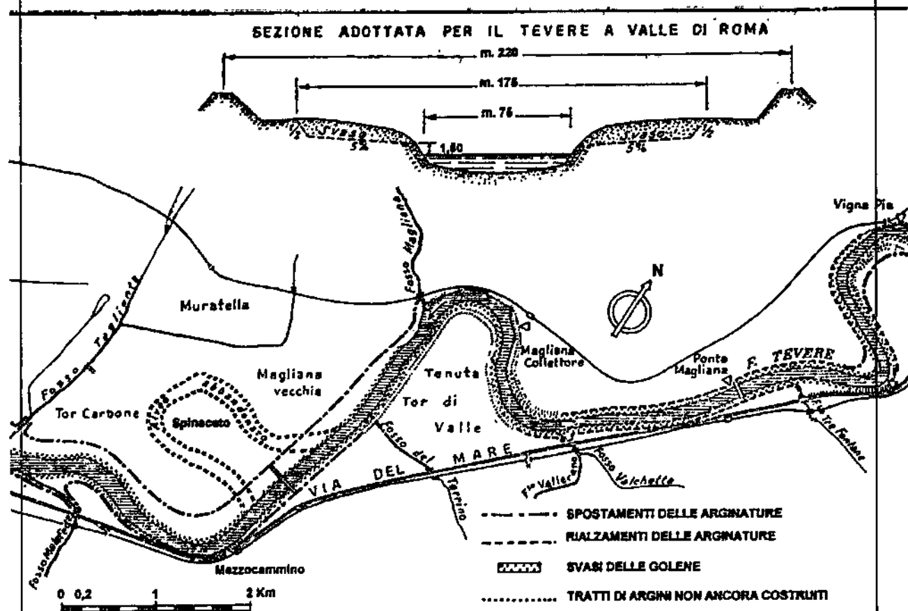
Fig. 2- Il meandro di Tor di Valle e il drizzaggio di Spinaceto. Il Fosso di Vallerano in sinistra idrografica del Tevere (Fonte: Frosini, 1977, modificato).
