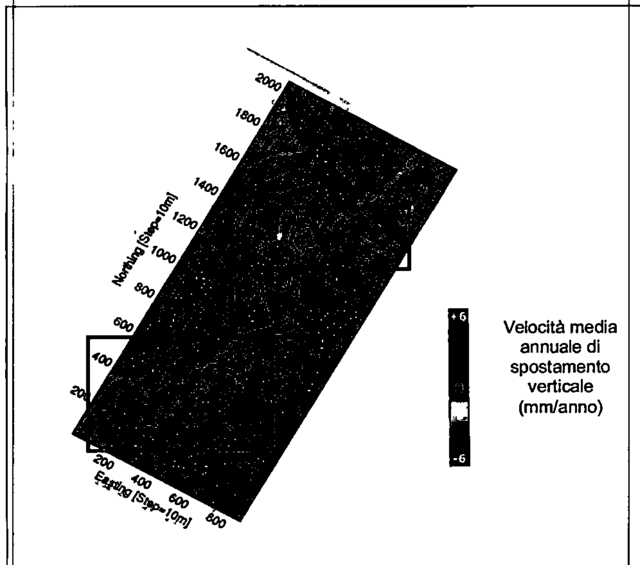
Fig. 3 – Il meandro nella parte inferiore della immagine è quello in esame. Come si nota, la velocità di subsidenza indicata dai rilievi interferometrici satellitari è pari ad almeno 3-4 mm/anno (Fonte: Campolunghi ed altri, 2008).
